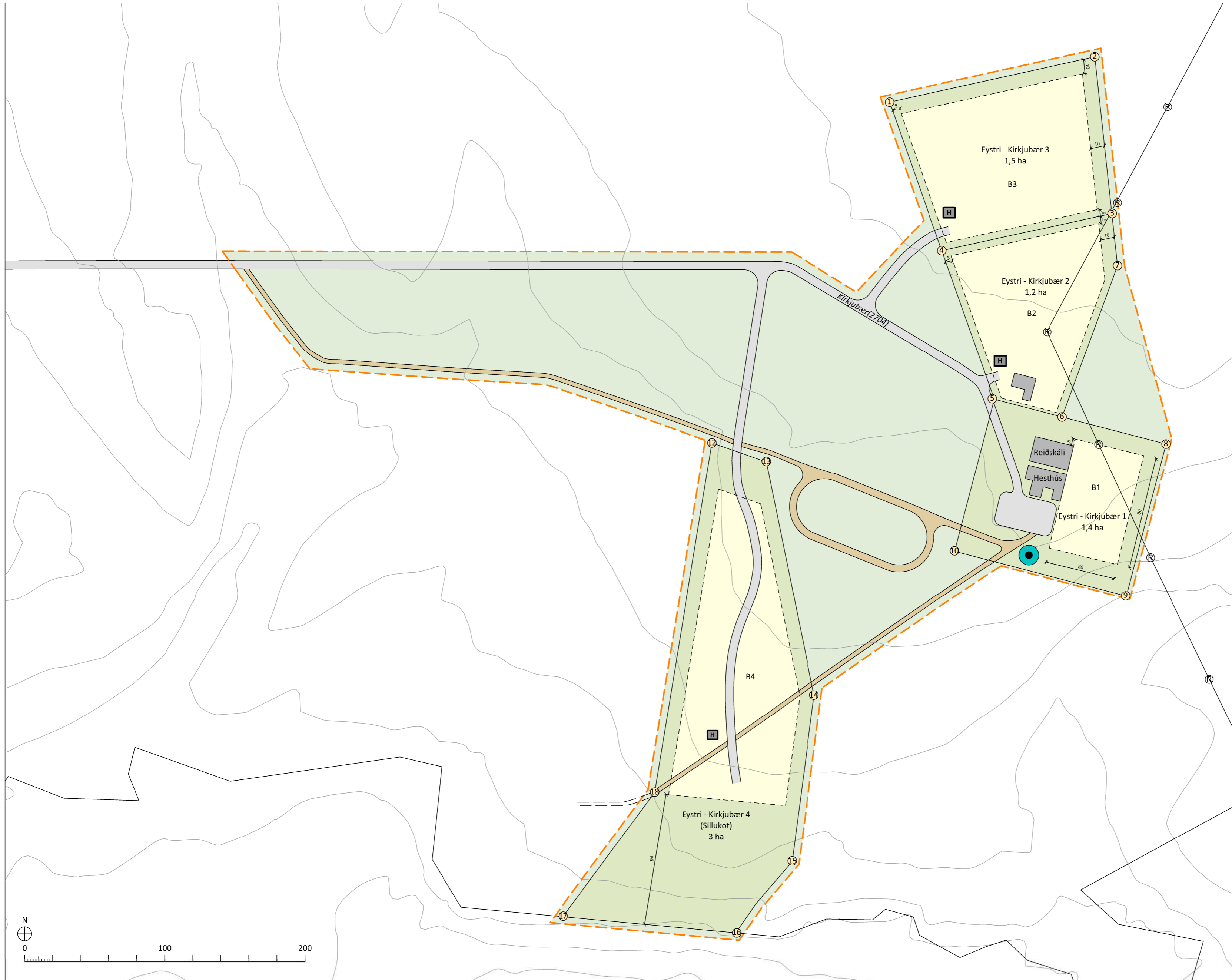
DEILISKIPULAGSUPPDRAÐTÚR 1:2000
